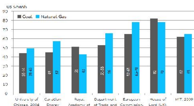
รูปที่ ๕ ต้นทุนเฉลี่ยตลอดอายุของโรงไฟฟ้า (Levelised cost) เทียบระหว่างถ่านหินกับก๊าซธรรมชาติ
