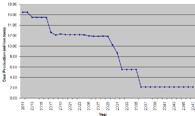
รูปที่ ๔ แผนการผลิตถ่านหินของเหมืองแม่เมาะ
