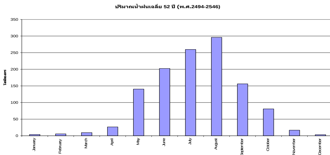
รูปที่ 4 ปริมาณน้ำฝนที่ตกในลุ่มน้ำแม่ตาบ เฉลี่ย 52 ปี (พ.ศ.2494-2546) (ปรับปรุงจากข้อมูลของบริษัท ผาแดงอินดัสทรี จำกัด (มหาชน))
