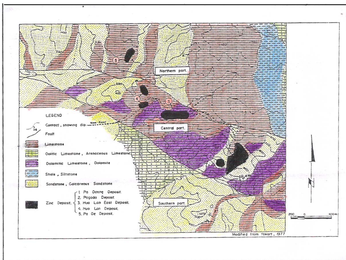
รูปที่ 3 แผนที่ธรณีวิทยาแหล่งแร่ของเหมืองแร่สังกะสี หมู่เหมืองคอยผาแดง อำเภอแม่สวด จังหวัดตาก
