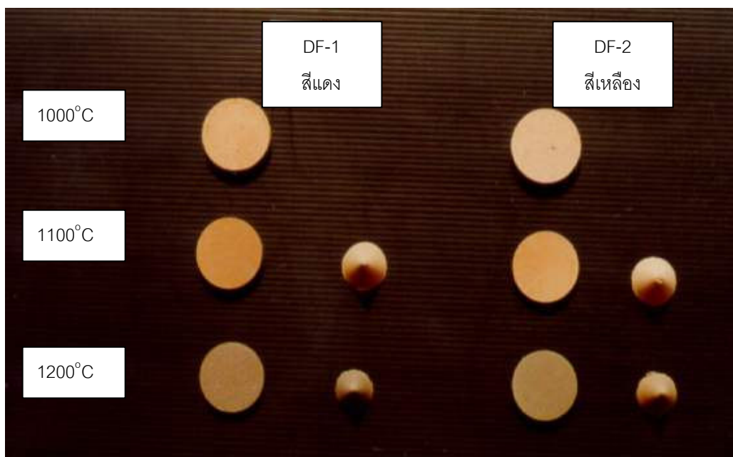
รูปที่ 4.5 แสดงสีของชิ้นงานตัวอย่างดินห้วยเสือ-ดอนไฟที่ผ่านการเผาที่ 1200°C
