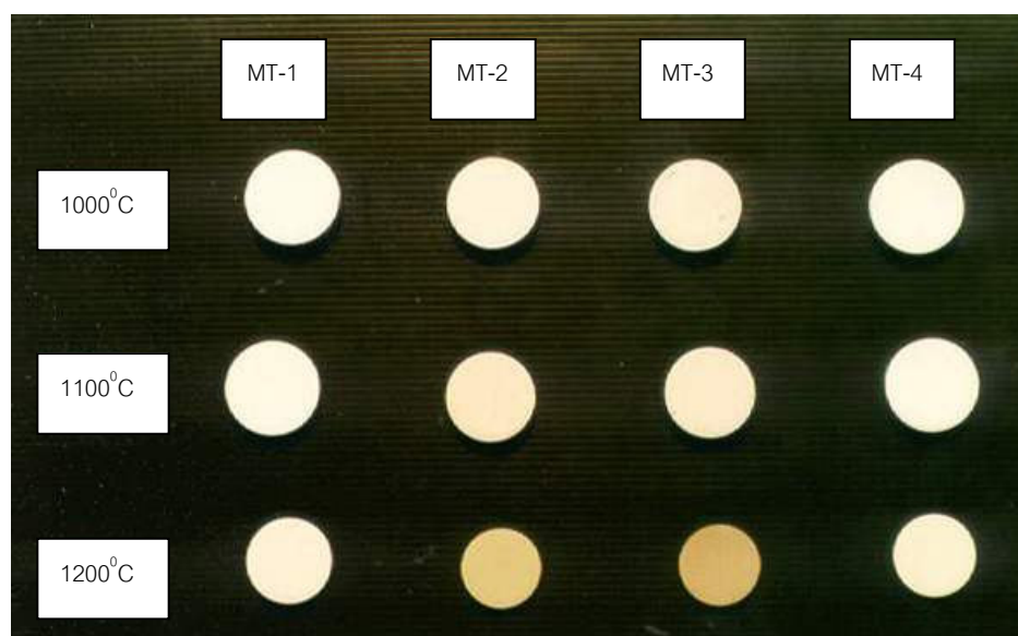
รูปที่ 4.3 แสดงการเปลี่ยนแปลงคุณลักษณะของดินแม่ทานที่อุณหภูมิการเผาที่ต่างกัน
