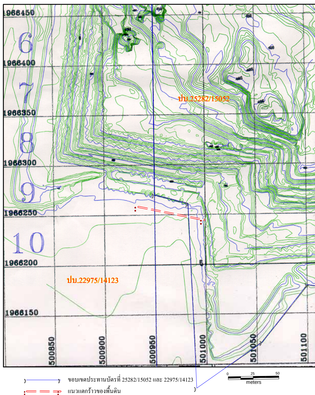
รูปที่ 6 แผนที่บริเวณขอบขุมเหมืองที่ปรากฏรอยแตกร้าของแผ่นดิน
