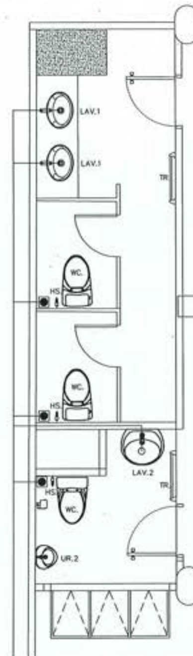
แบบระบบน้ำทิ้ง
