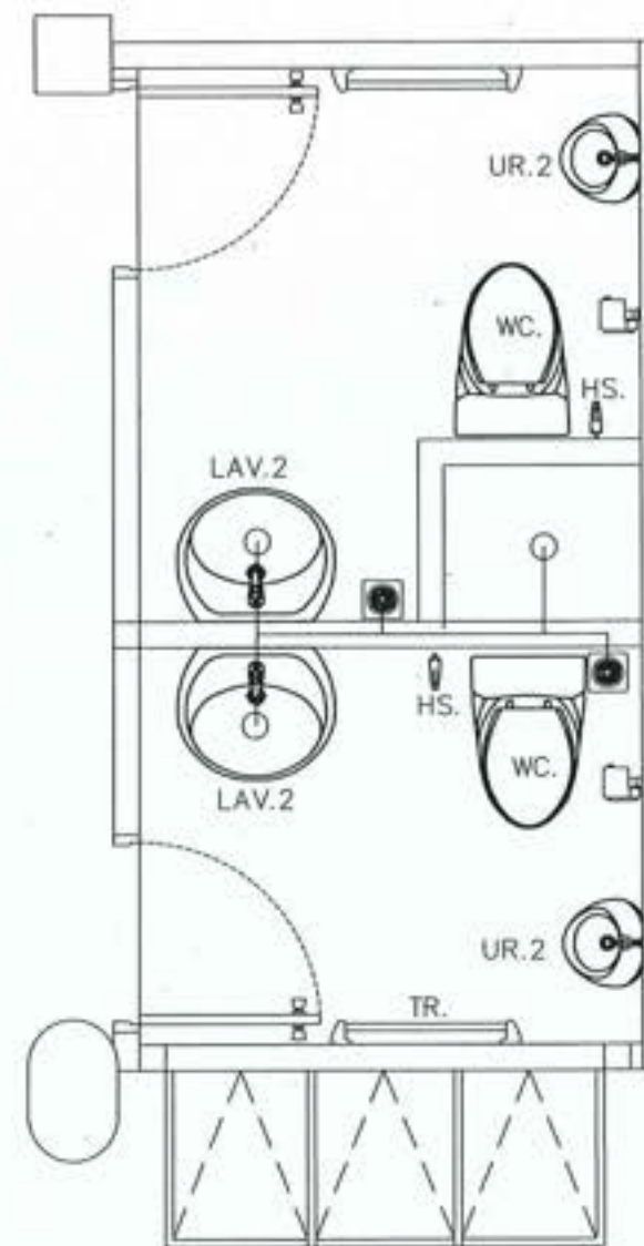
แบบระบบน้ำทิ้ง
