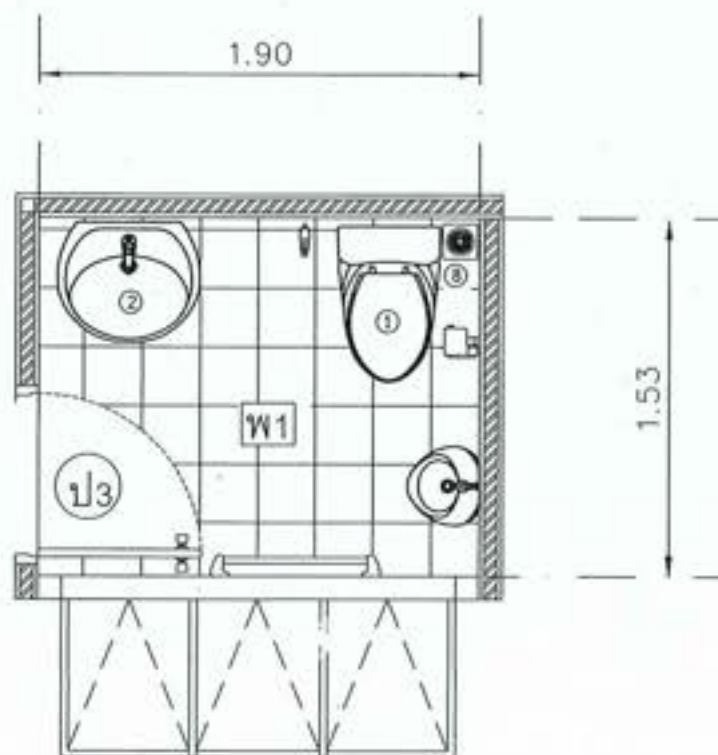
แปลนห้องน้ำ
