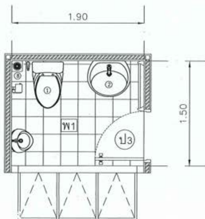
แปลนห้องน้ำ
