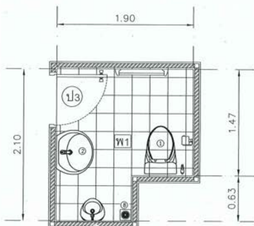
แปลนห้องน้ำ
