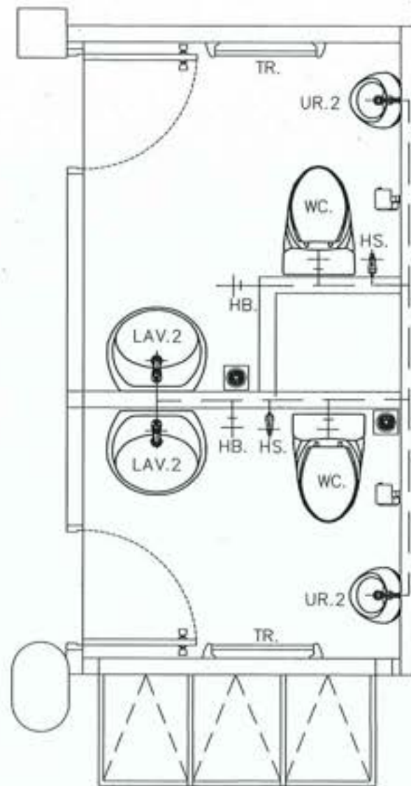
แบบระบบน้ำดี
