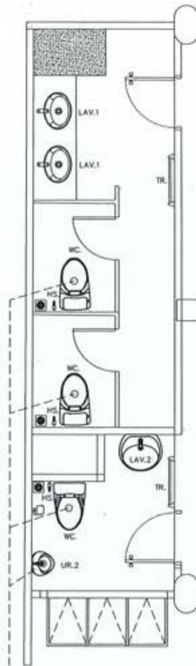
แบบระบบน้ำเสีย
