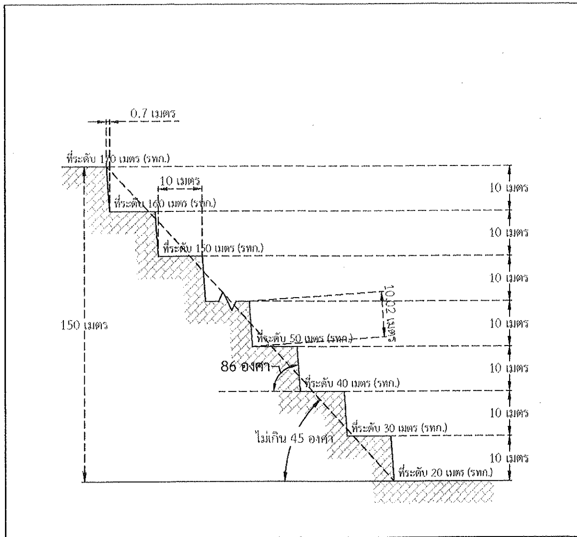
รูปที่ 2. ภาพแสดงการทำเหมืองแบบขั้นบันได
